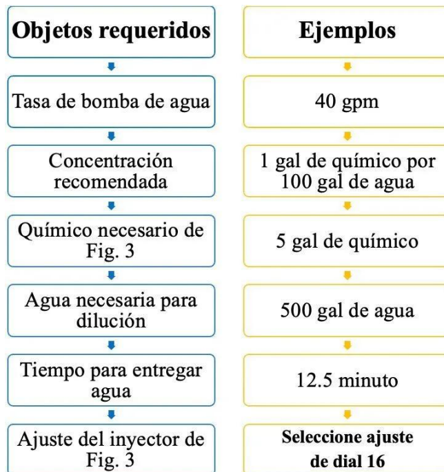
Figura 3. Ejemplo de pasos para determinar el ajuste apropiado de inyector. Los pasos para el cálculo de la cantidad de producto químico necesario se muestran anterior en la Figura 2.
